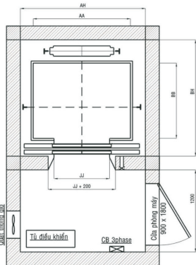
THANG TẢI KHÁCH ĐỐI TRỌNG PHÍA SAU
