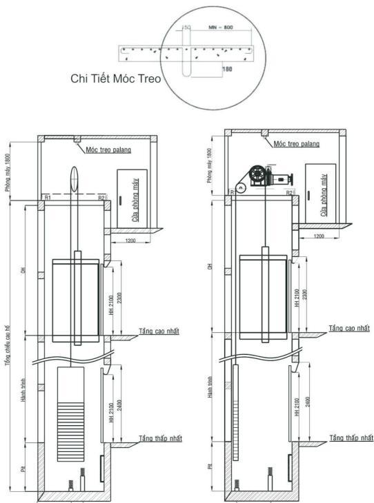
THANG TẢI KHÁCH ĐỐI TRỌNG BÊN HÔNG
