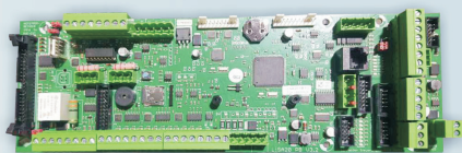
Bộ vi xử lý LISA20 (DLR LISA20 PB)
