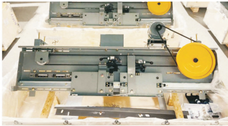
Đầu cửa cabin
