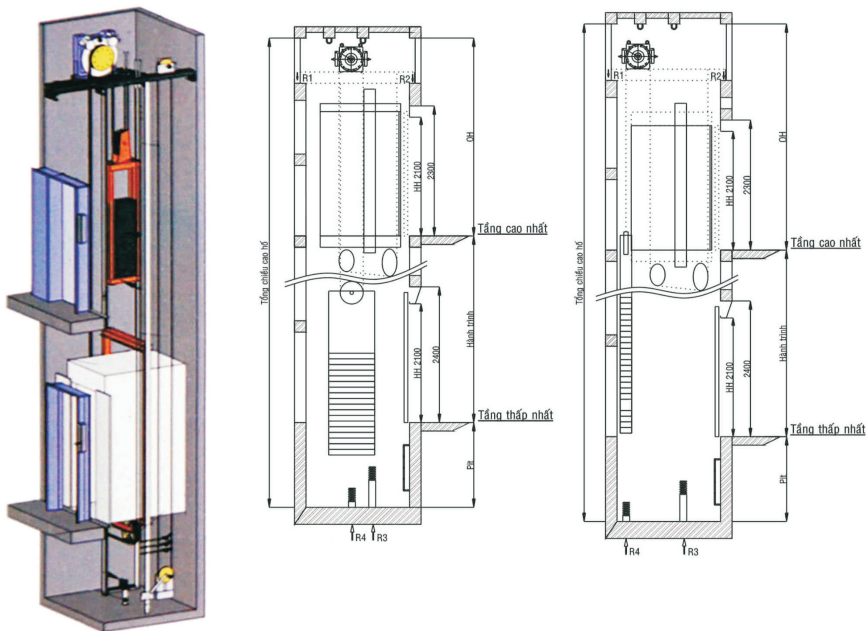
THANG TẢI KHÁCH ĐỐI TRỌNG PHÍA SAU
