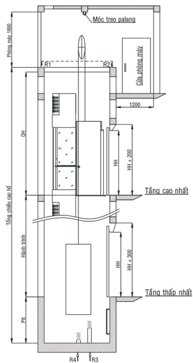
THANG CÓ PHÒNG MÁY
