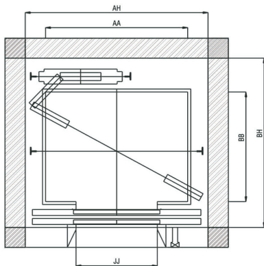
THANG TẢI KHÁCH ĐỐI TRỌNG PHÍA SAU
