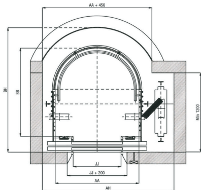
THANG KHÔNG PHÒNG MÁY
